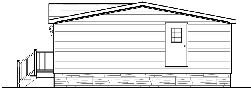
RIGHT ELEVATION
